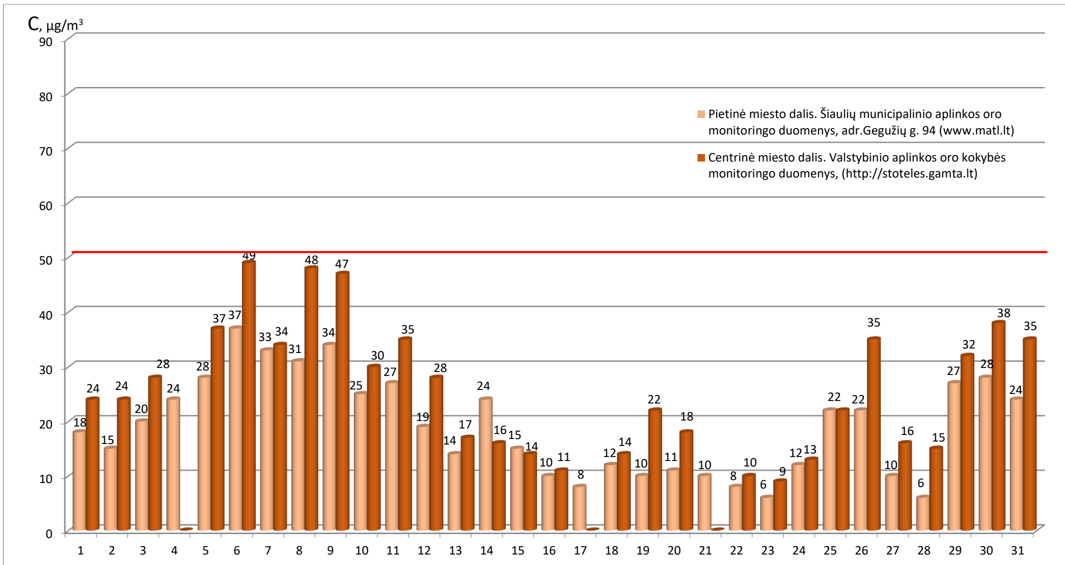
1 pav. Kietųjų dalelių (KD 10 ) vidutinės 24 val. koncentracijos kitimas Šiaulių m. aplinkos ore 2021 m. spalio 1 ÷ 31 d. (Ribinė vertė 50 µg/m 3 ).
